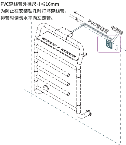
暗装设备连接图示：
