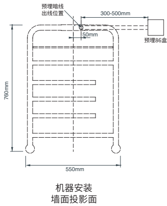
预埋出线位置图示：
