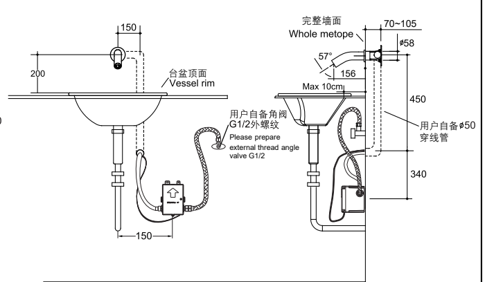
欧宝入墙式单冷直流感应龙头
