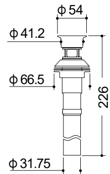
Drain 排水组件
