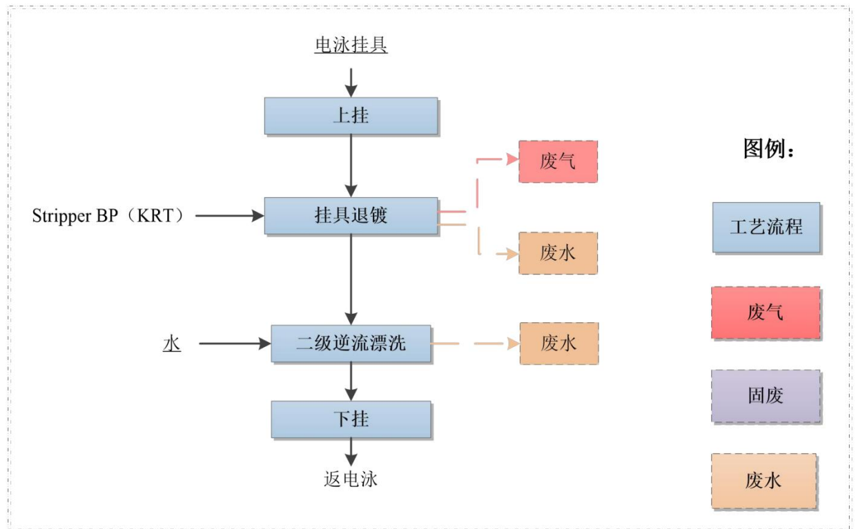
图 3-14 电泳挂具褪镀工艺流程及产污节点图 工艺流程简述：
