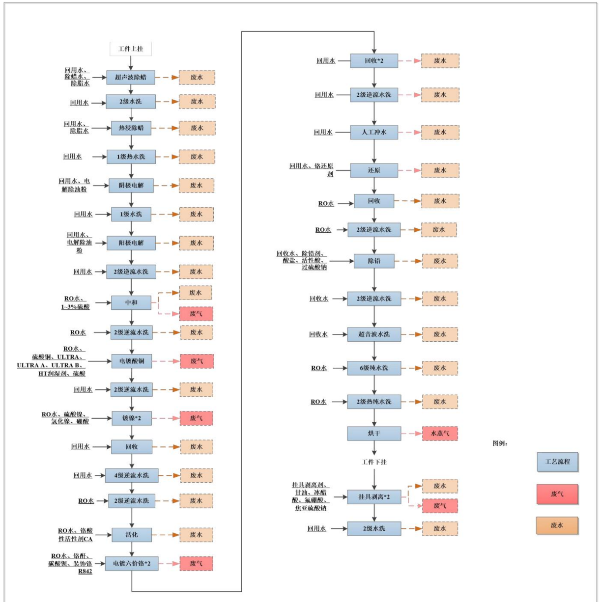
图 3-8 电镀铬生产线工艺流程及产污节点图 电镀铬生产线生产工艺与前述两条电镀线基本一致。
