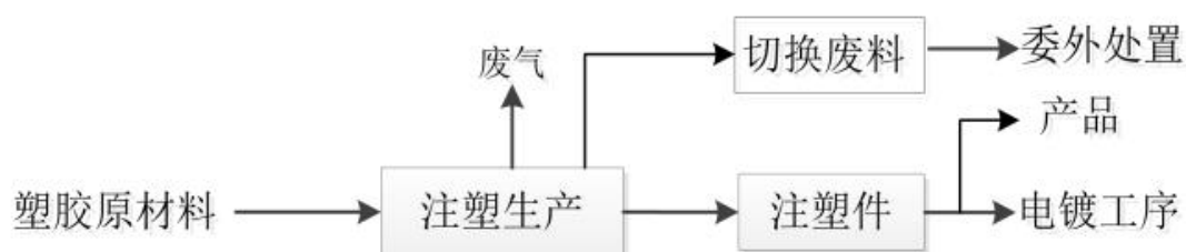
图 3-16 塑料花洒项目注塑工艺流程及产污节点图
