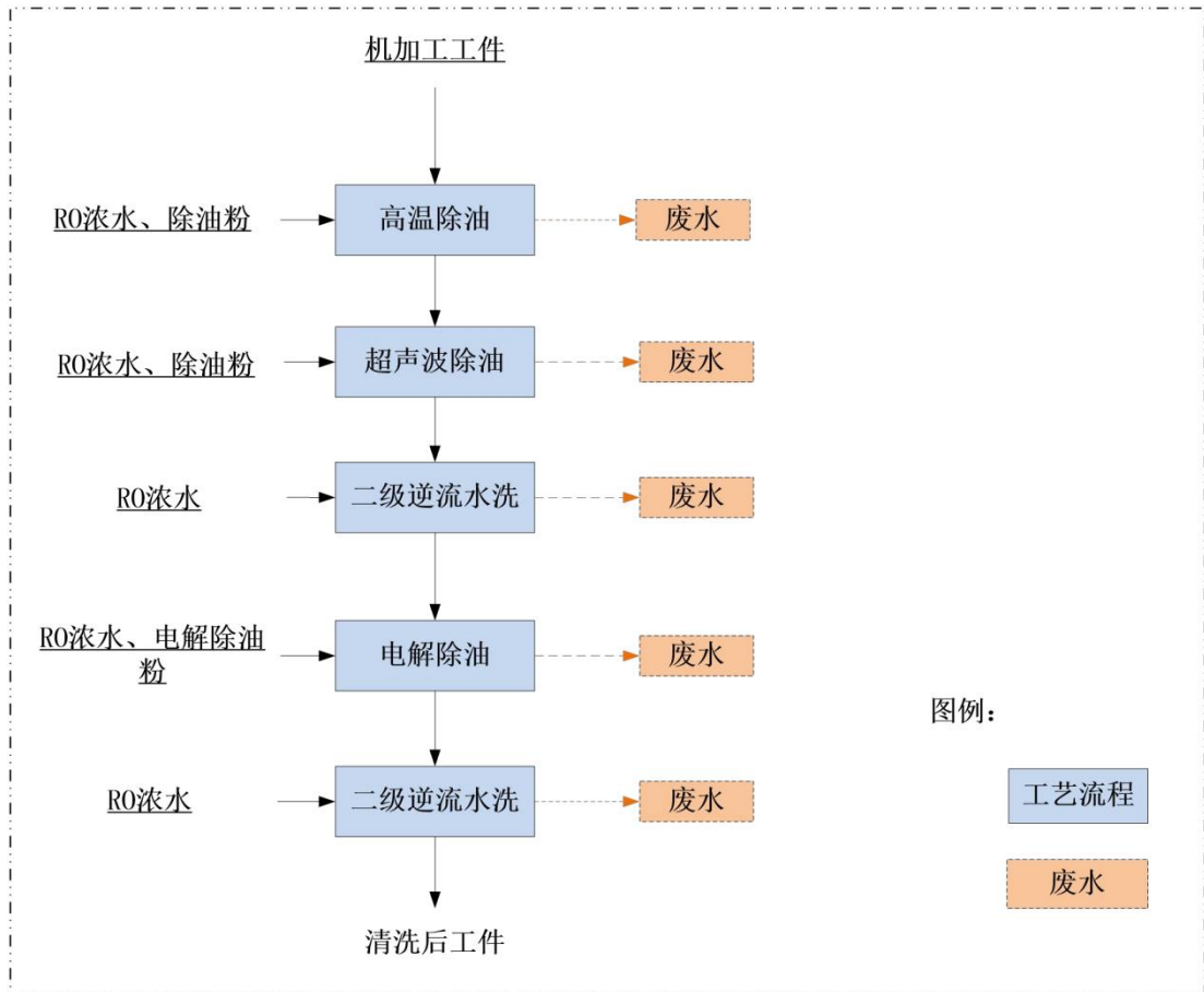
图 3-3 机加工清洗线工艺流程图
