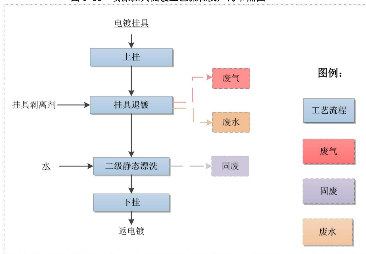
图 3-12 电镀挂具褪镀工艺流程及产污节点图
