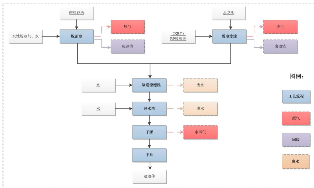
图 3-15 退漆工艺流程及产污节点图
