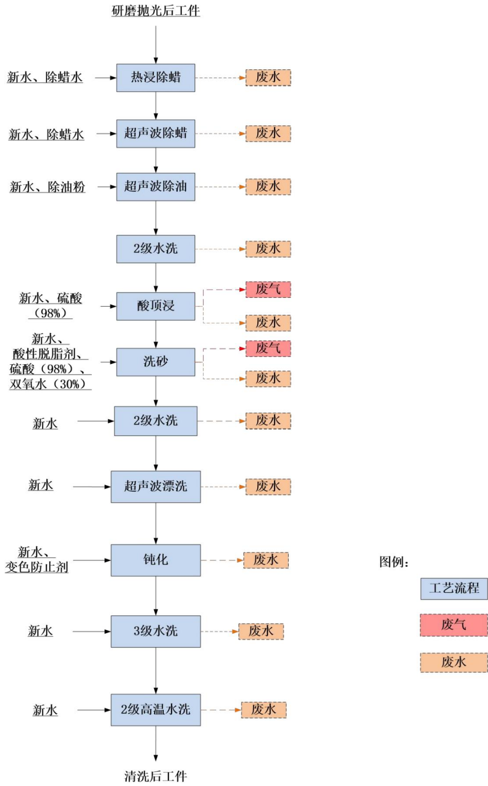
图 3-4 研磨抛光清洗线工艺流程图
