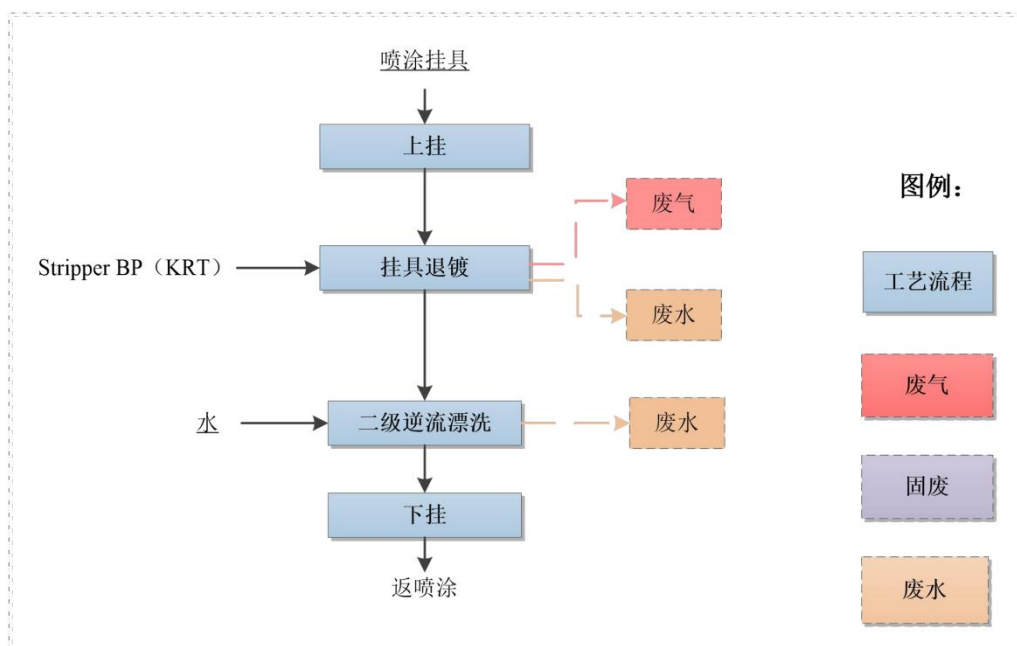
图 3-11 喷涂挂具褪镀工艺流程及产污节点图
