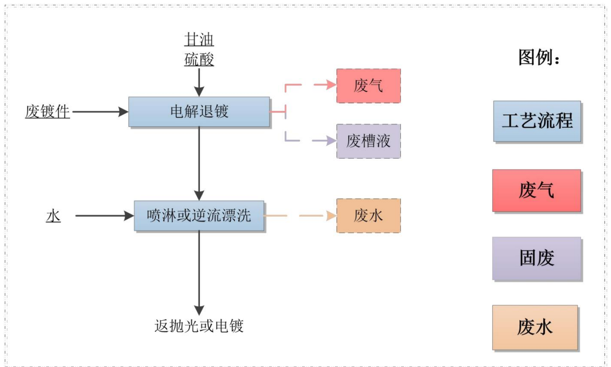
图 3-9 褪镀工艺流程及产污节点图 褪镀后的工件返回相应的抛光工序或电镀生产线。
