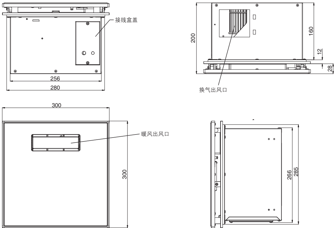
产品尺寸图 (单位：毫米)
