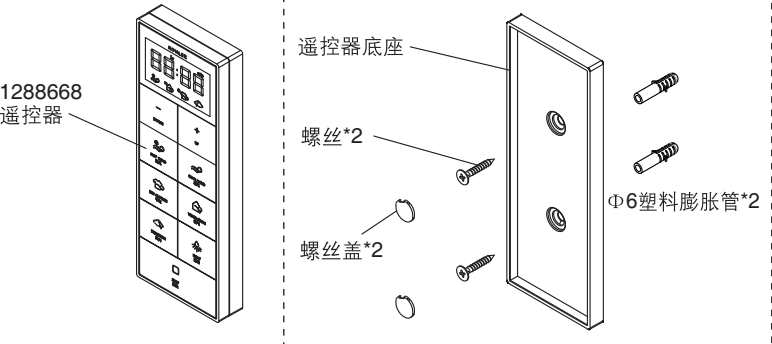
1285556 遥控器底座组件
