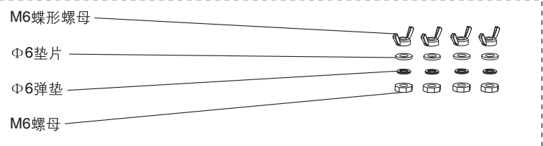
1285553 锁紧组件
