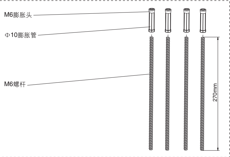
1285553 锁紧组件
