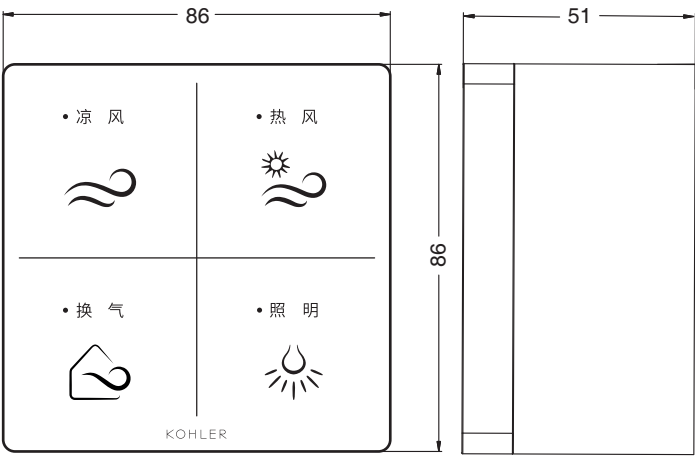
墙装开关尺寸图
