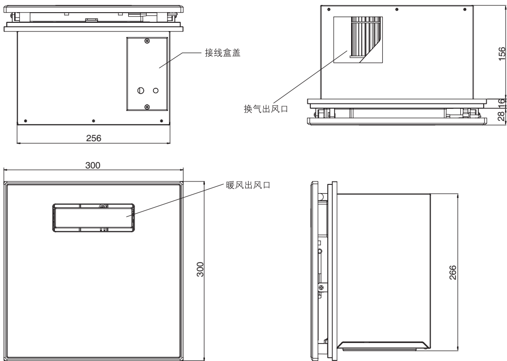
产品尺寸图 (单位：毫米)
