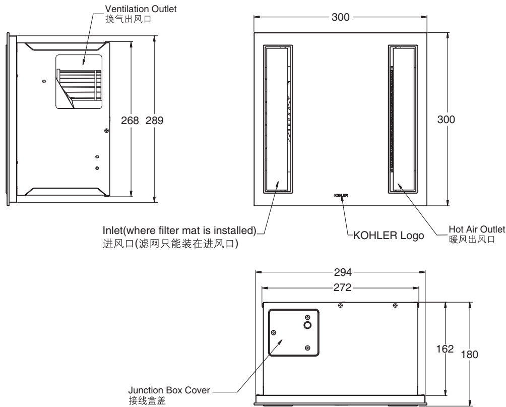
ROUGHING-IN 产品尺寸图 (Unit:mm)(单位：毫米)
