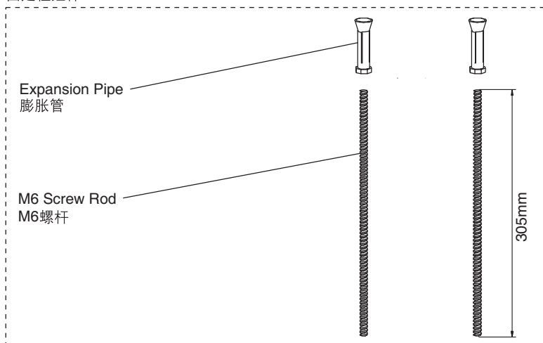
1322379 Fixed Column Assy. 固定柱组件
