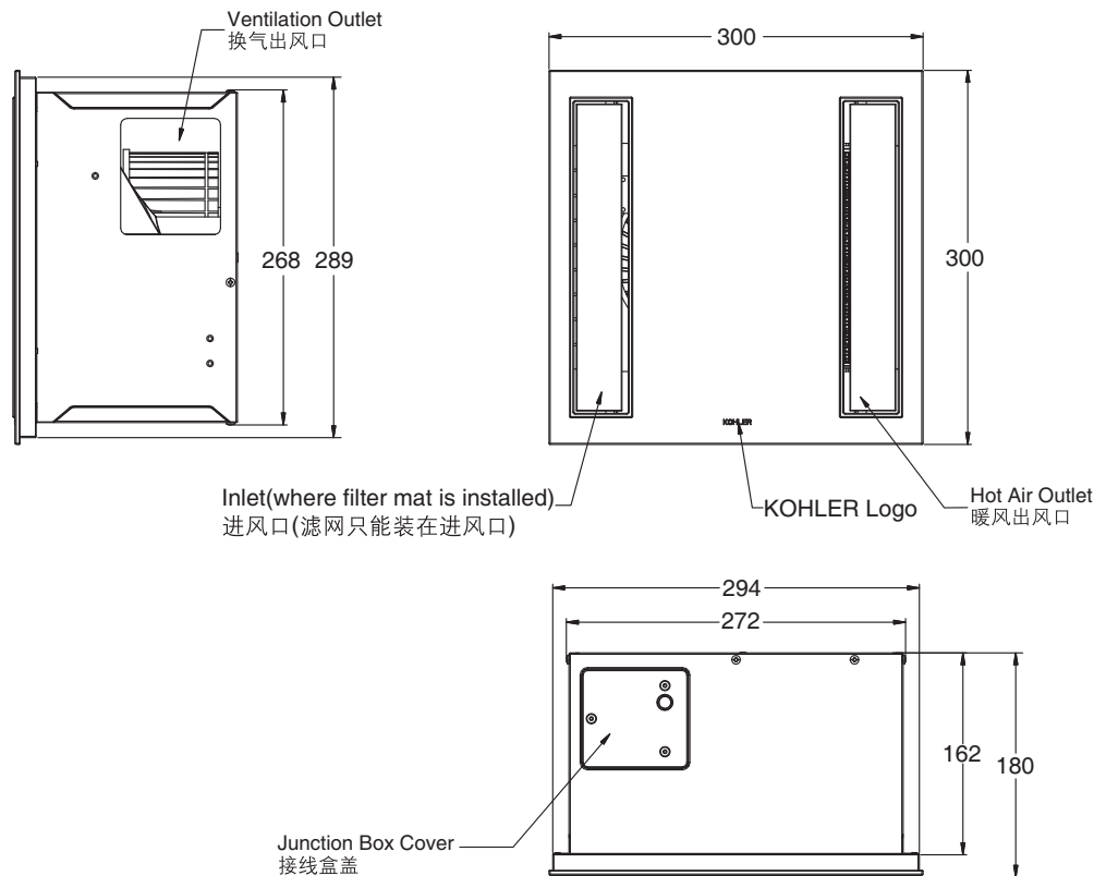
ROUGHING-IN 产品尺寸图 (Unit:mm)(单位：毫米)
