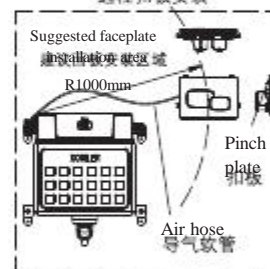
Method four: Press from front 安装方式四 前按扣板安装
