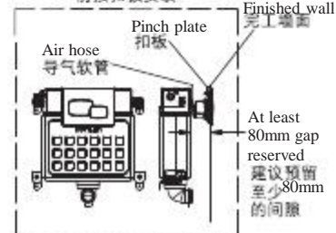
Method four: Press from front 安装方式四 前按扣板安装
